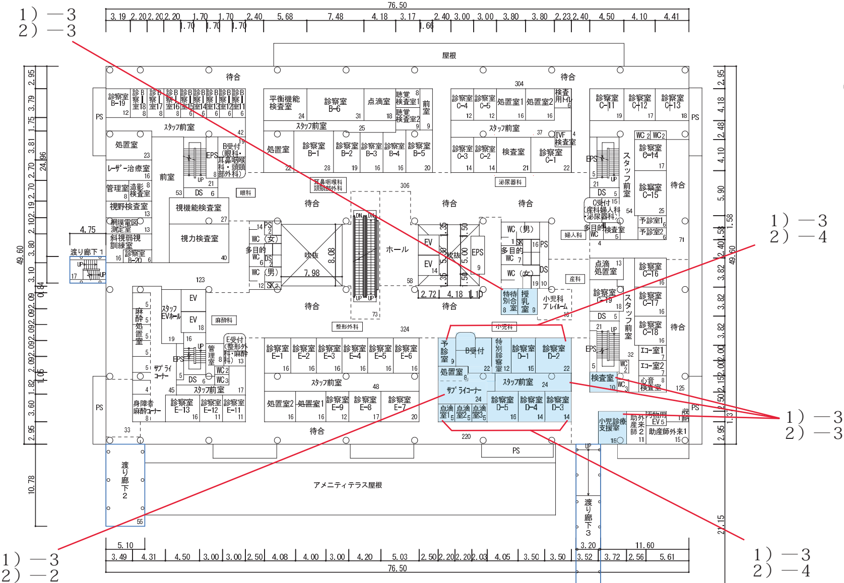
2階平面図 S = 1 / 500 (3,825㎡)
