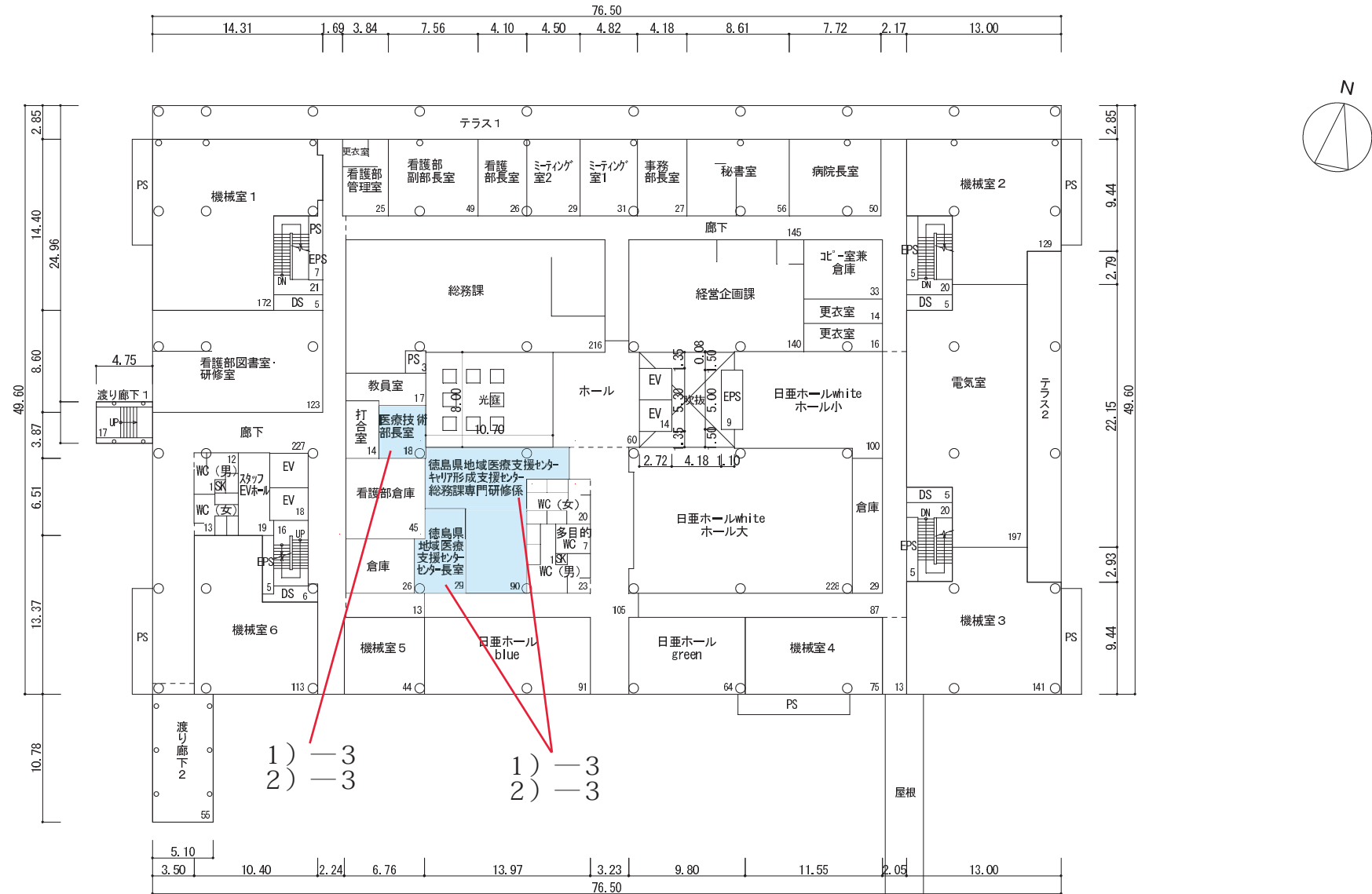
5 階平面図
