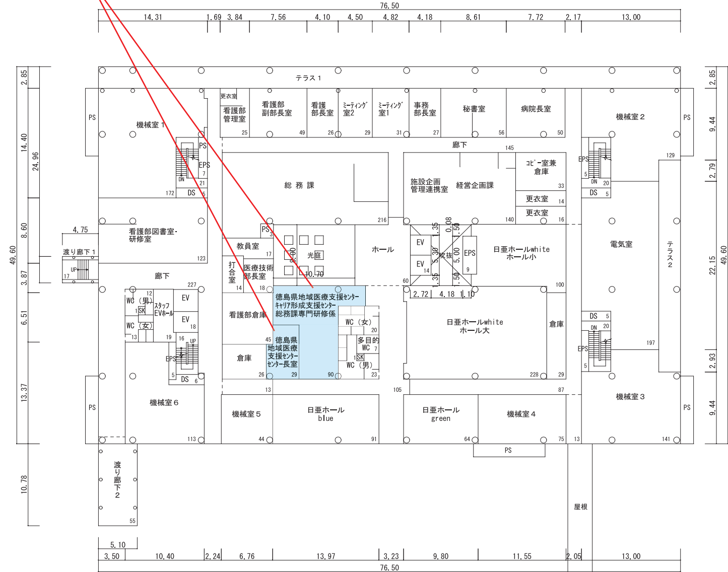
5 階 平 面 図 s = 1 / 5 0 0 (3,439㎡) (実 態 用 : 3,404㎡)
