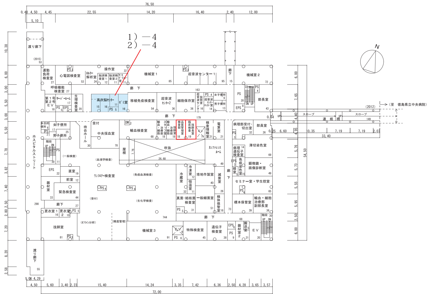
3 階 平 面 図 s = 1/600 (4,231㎡) (実態用 : 4,149㎡)
