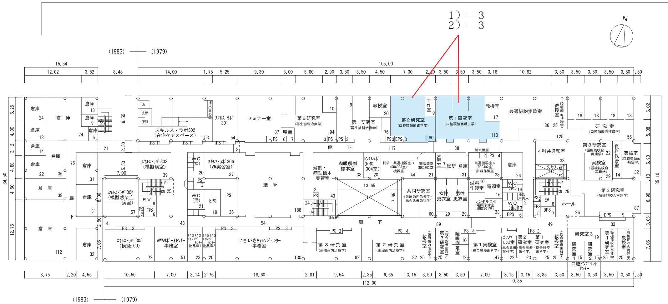
3階平面図 S = 1 / 500 (4,267㎡)
