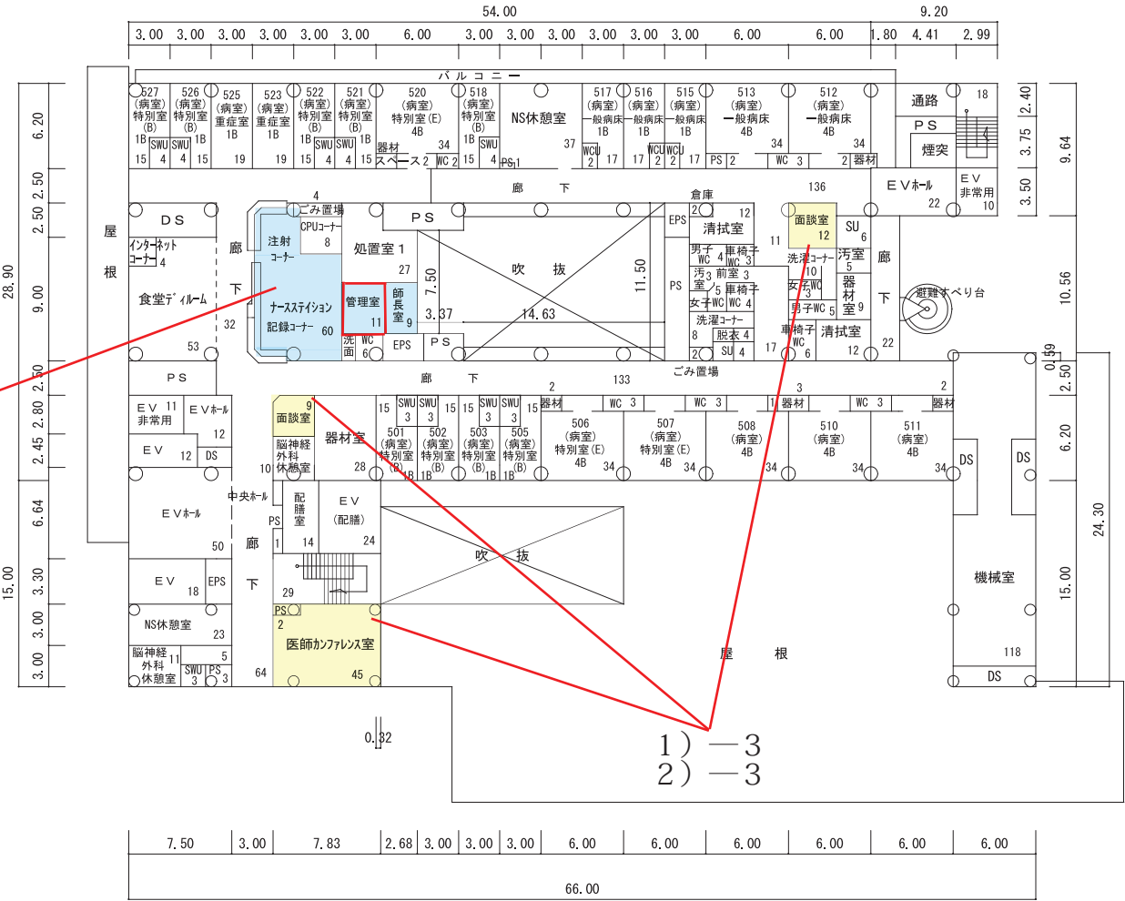
5 階平面図 S=1/500 (1998- 1,797㎡) (1,797㎡～実態用)
