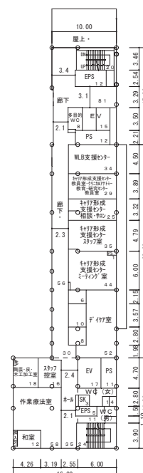
4 階平面図 (702m 2 )
