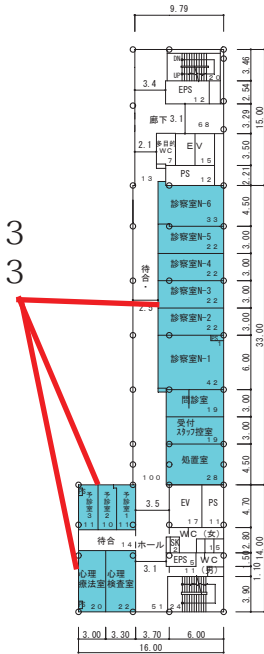
5 階平面図 (701m 2 )
