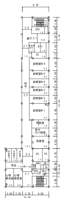
5 階平面図 (701m 2 )
