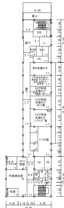
4 階平面図 (702m 2 )
