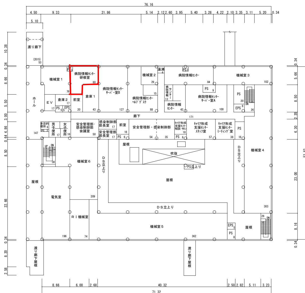
5 階 平 面 図 s = 1/600 (2,881 m^2 ) (実態用 : 946 m^2 )
